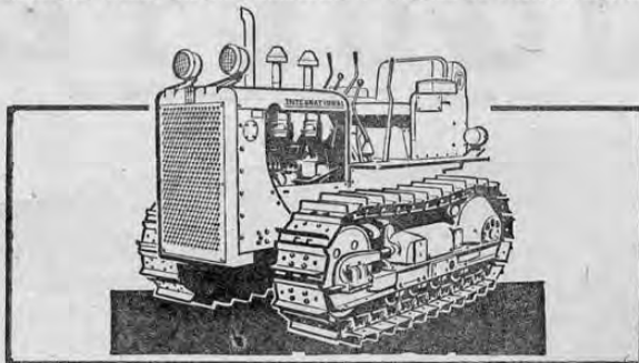
Modelo BTD-8 de orugas equipado con pala y winch Motor Diesel de 60 caballos, 4 cilindros a 1.600 R. P. M.
